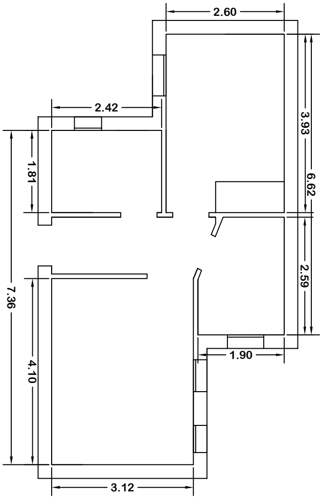
Plano acotado
